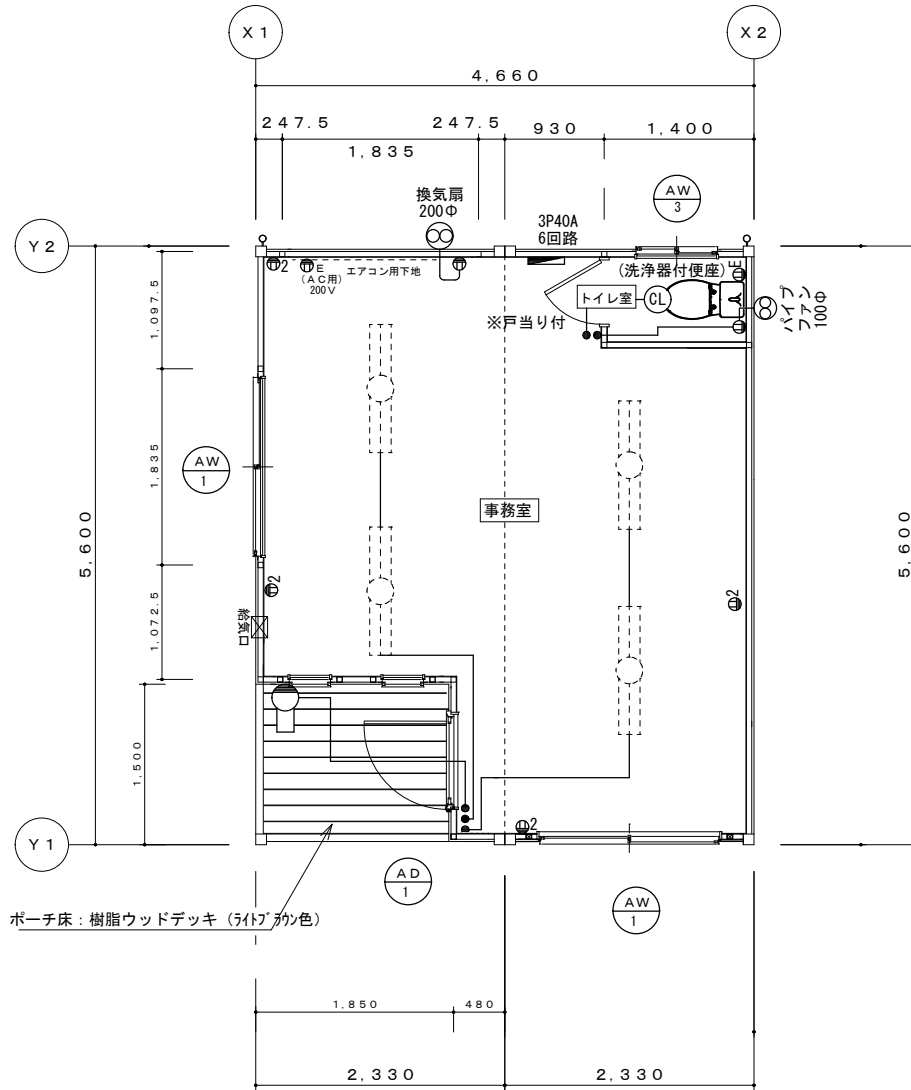
平面図 S = 1/50
