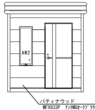
X2立面図 S=1/50
