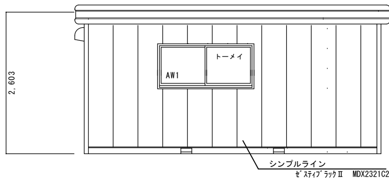
Y1立面図 S=1/50
