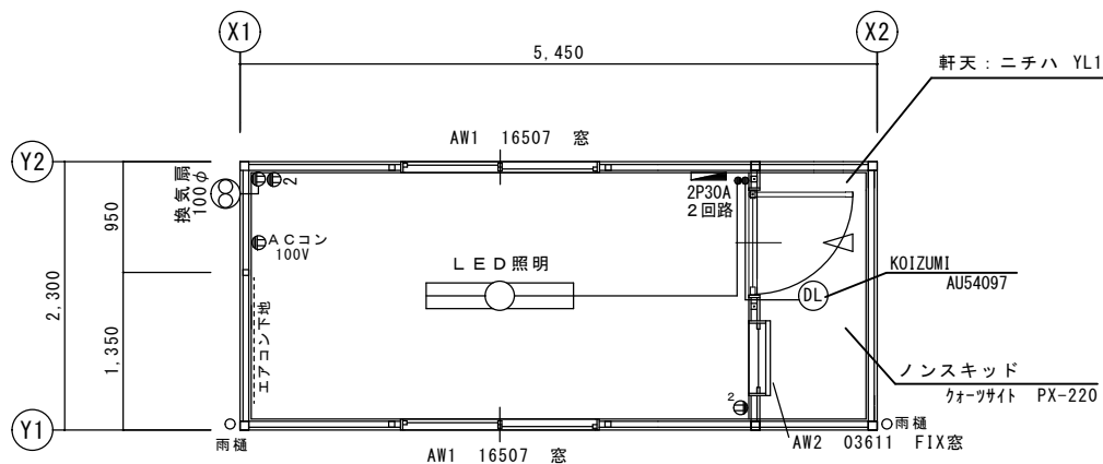
平面図 S=1/50
