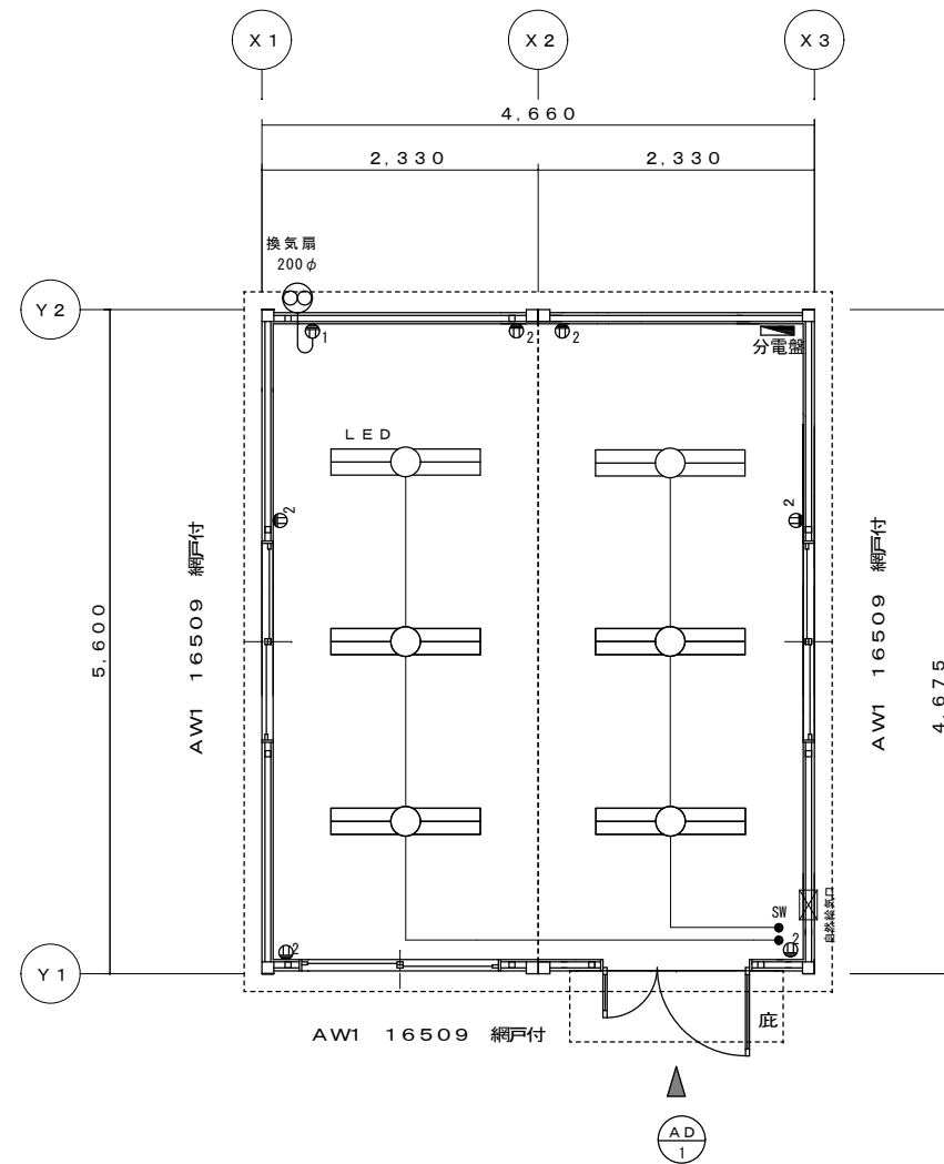
平面図 S = 1/50
