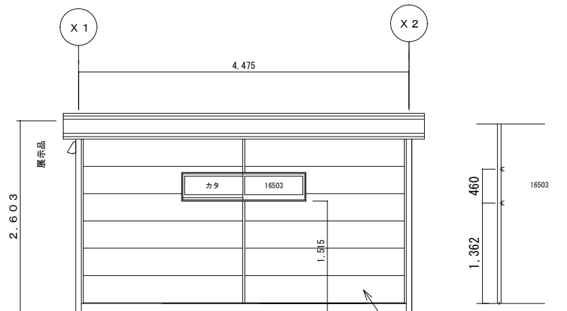
Y2 立面図
