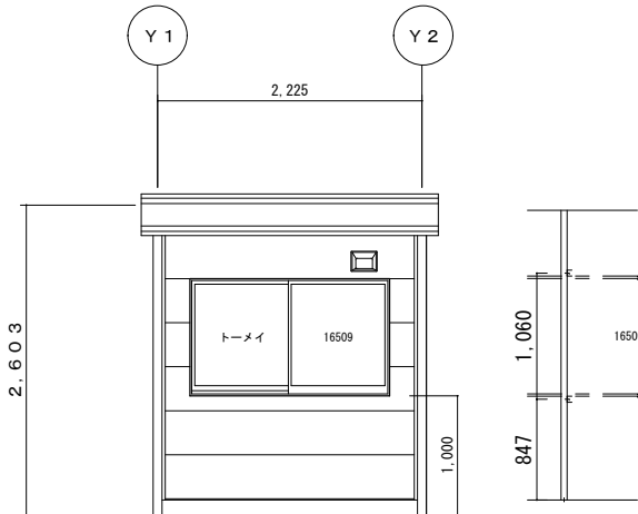
X2 立面図
