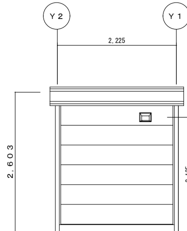
X1 立面図
