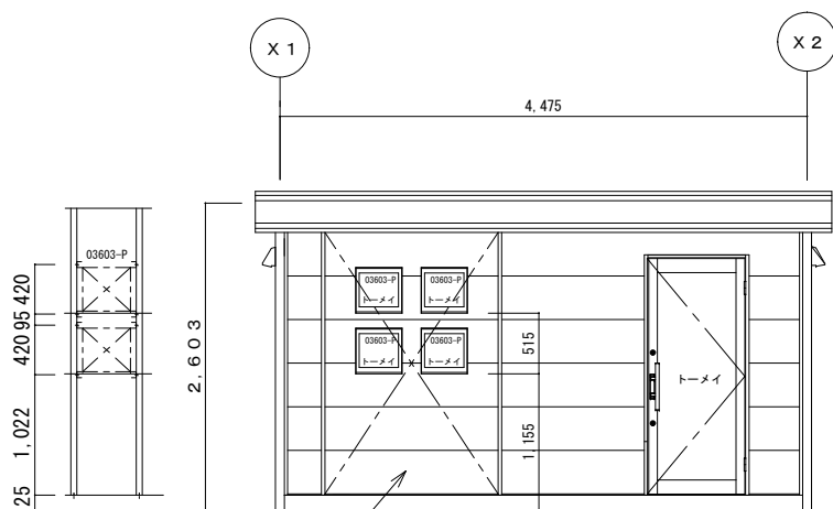
Y1 立面図
