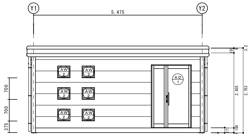
X1側立面図 S = 1 / 5 0
