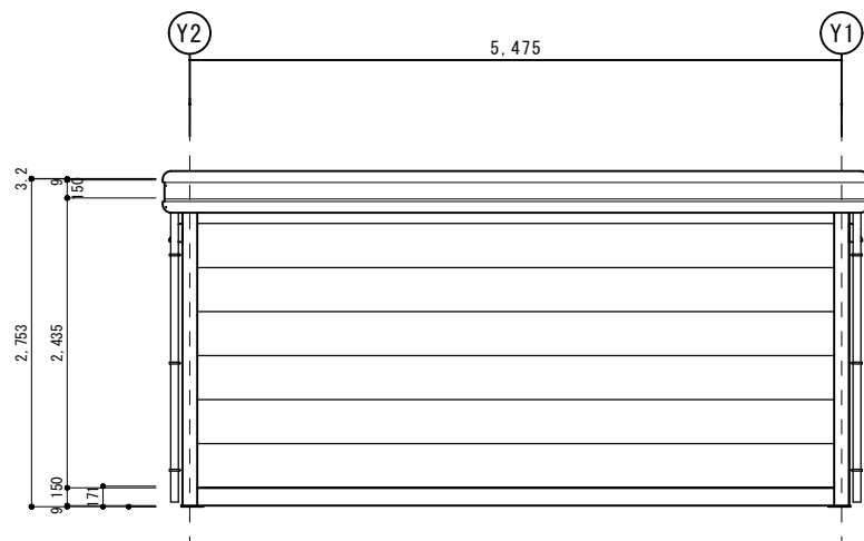
X2側立面図 S = 1 / 5 0
