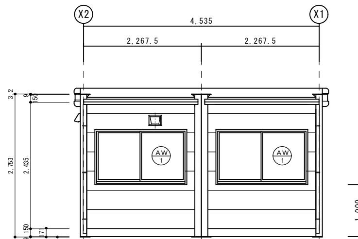
Y1側立面図 S = 1 / 50
