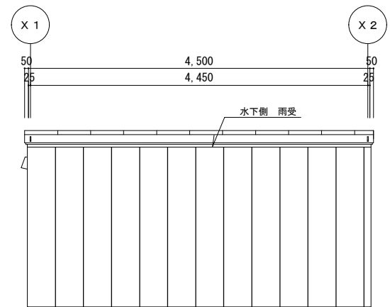
Y 1 立面図 S=1/50
