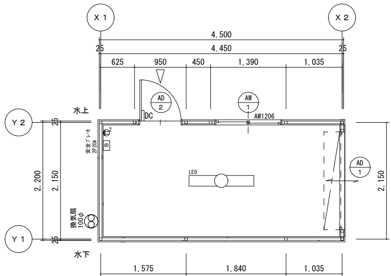
平面図 S=1/50
