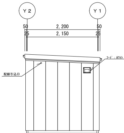
X 1 立面図 S=1/50
