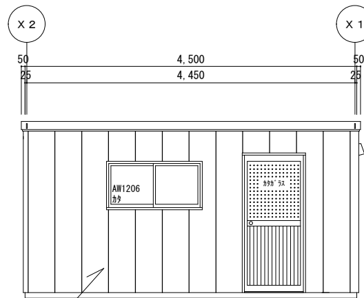
Y 2 立面図 S=1/50
