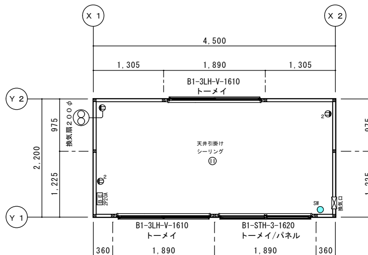
平面図 S=1/50
